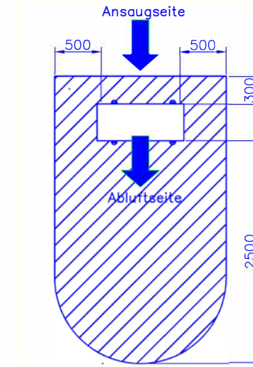
Aufstellhinweis
