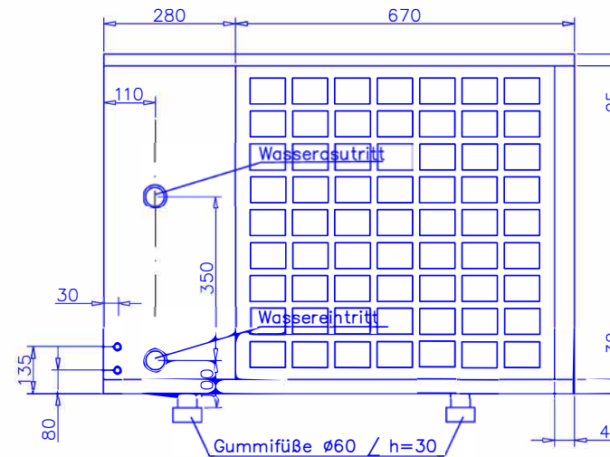
Rückansicht
