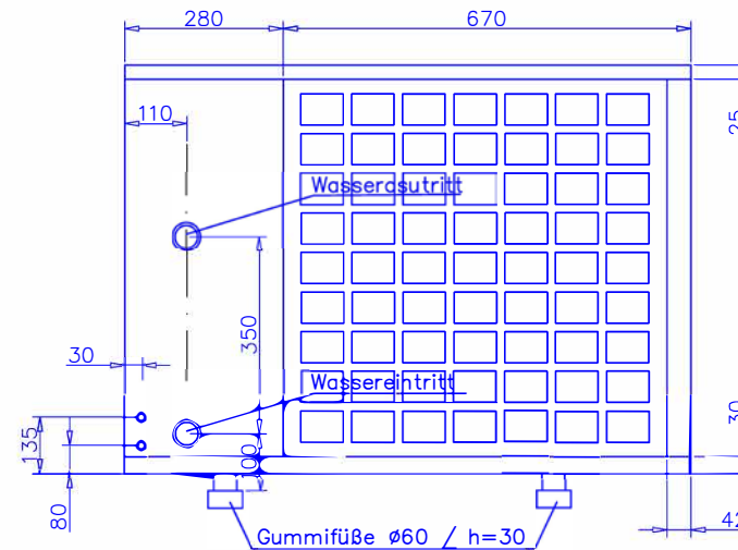
Rückansicht
