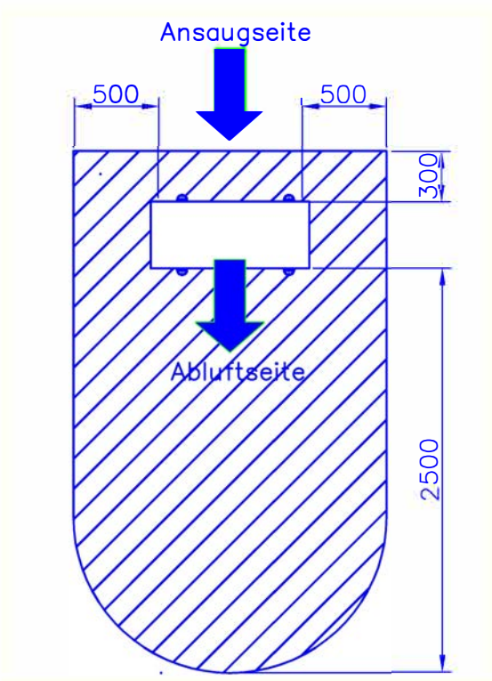
Aufstellhinweis
