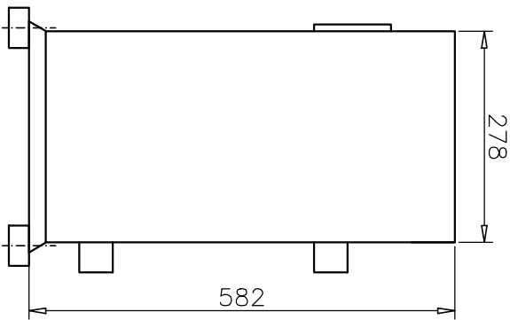
Draufsicht
