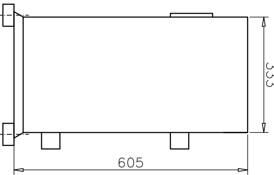
Vorderansicht
