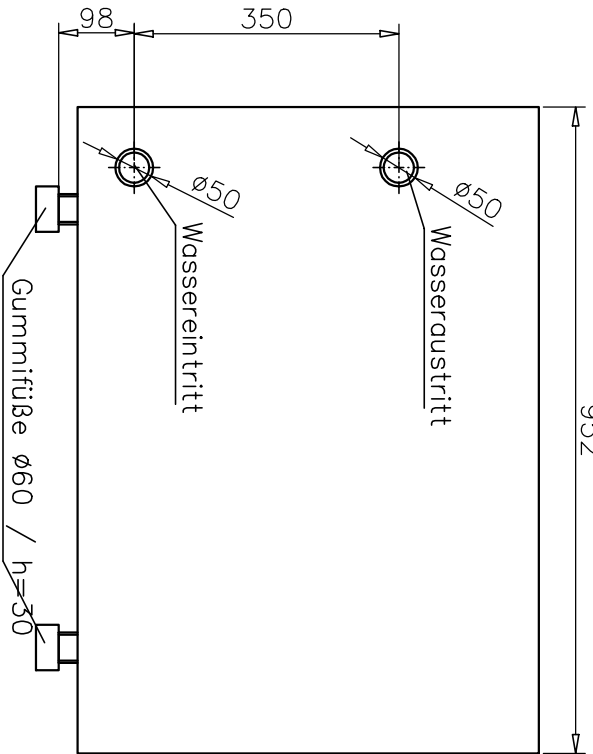
Seitenansicht von rechts
