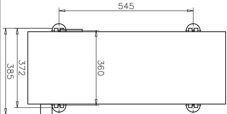
Draufsicht
