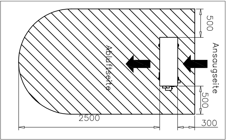
Aufstellhinweis
