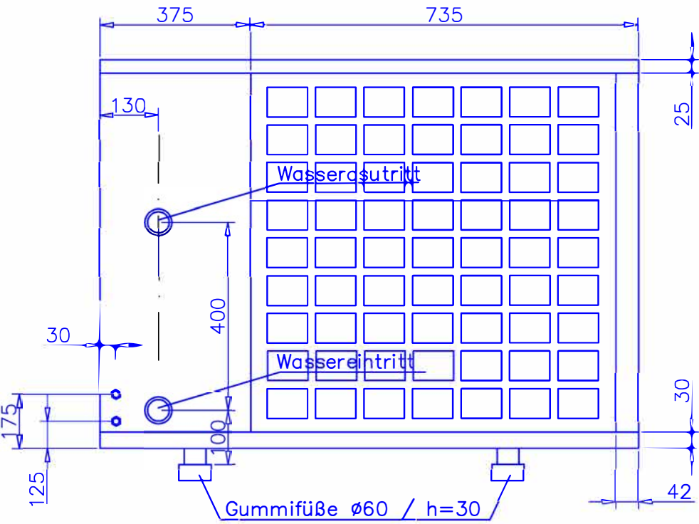
Rückansicht
