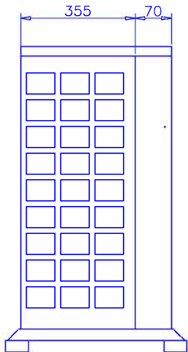
Seitenansicht von links
