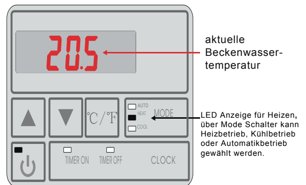
Betrieb LED (AN)
