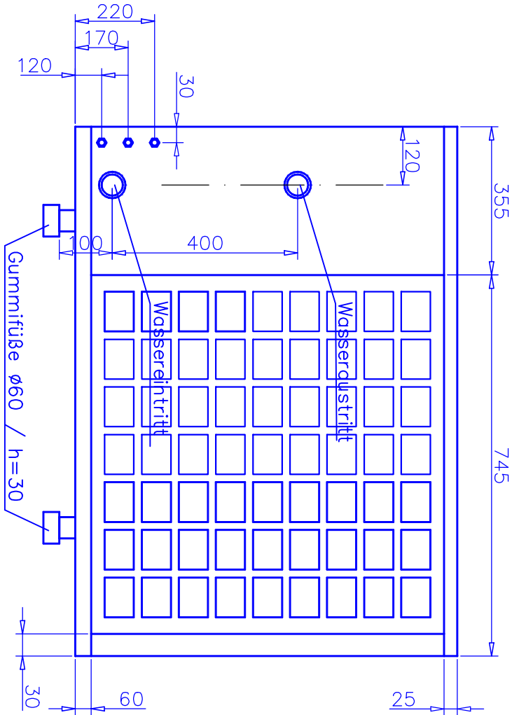
Rückansicht
