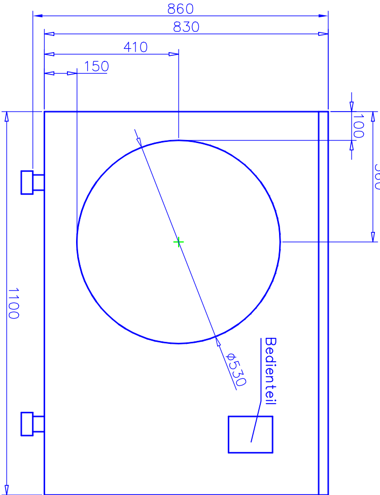
Vorderansicht
